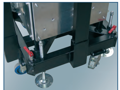
Stabilisateur renforcé M20
